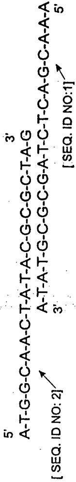
FIG. 4 Linking oligonucleotide
